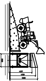
Ansicht Z
