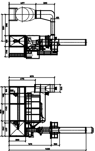
Schnitt E-E
